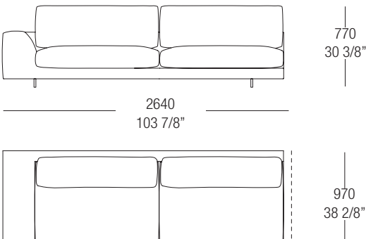
AG23TLD/S cuscino seduta diviso. split sitting cushion.
