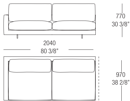
AG19TSD/S cuscino seduta diviso. split sitting cushion.
