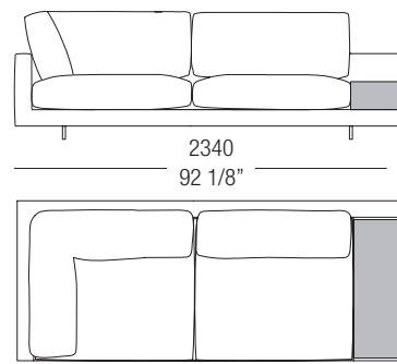
AG19AED/S cuscino seduta diviso. split sitting cushion.
