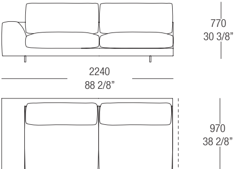
AG19TLD/S cuscino seduta diviso. split sitting cushion.
