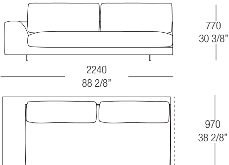
AG19TLUD/S cuscino seduta intero. full sitting cushion.
